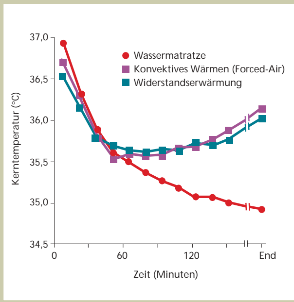
Abbildung 7: Effektivität von Wasser-, Luft- und Resistive-Heating-Systemen [9]
