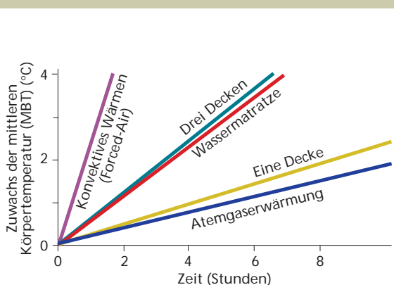
Abbildung 8: Effizienzvergleich verschiedener Wärmemethoden (Temperaturzuwachs pro Zeiteinheit)
